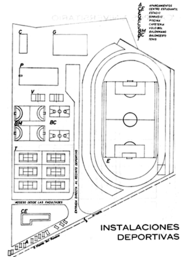
CEU. Plànol del projecte d'instal·lacions esportives. Font: Centre d'Estudis Universitaris d'Alacant. Elx, 1970 CEU. Plano del proyecto de instalaciones deportivas. Fuente: Centro de Estudios Universitarios de Alicante. Elche, 1970
